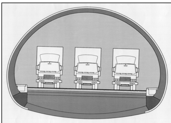
TYPICKÝ PŘÍČNÝ ŘEZ
