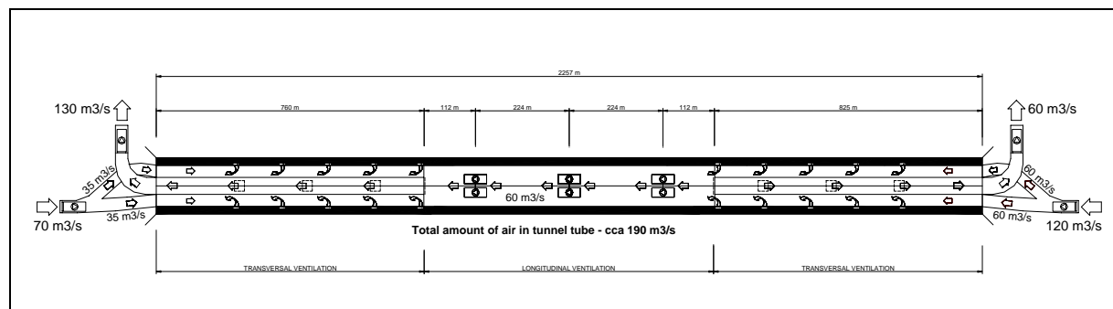
SCHÉMA VĚTRÁNÍ
